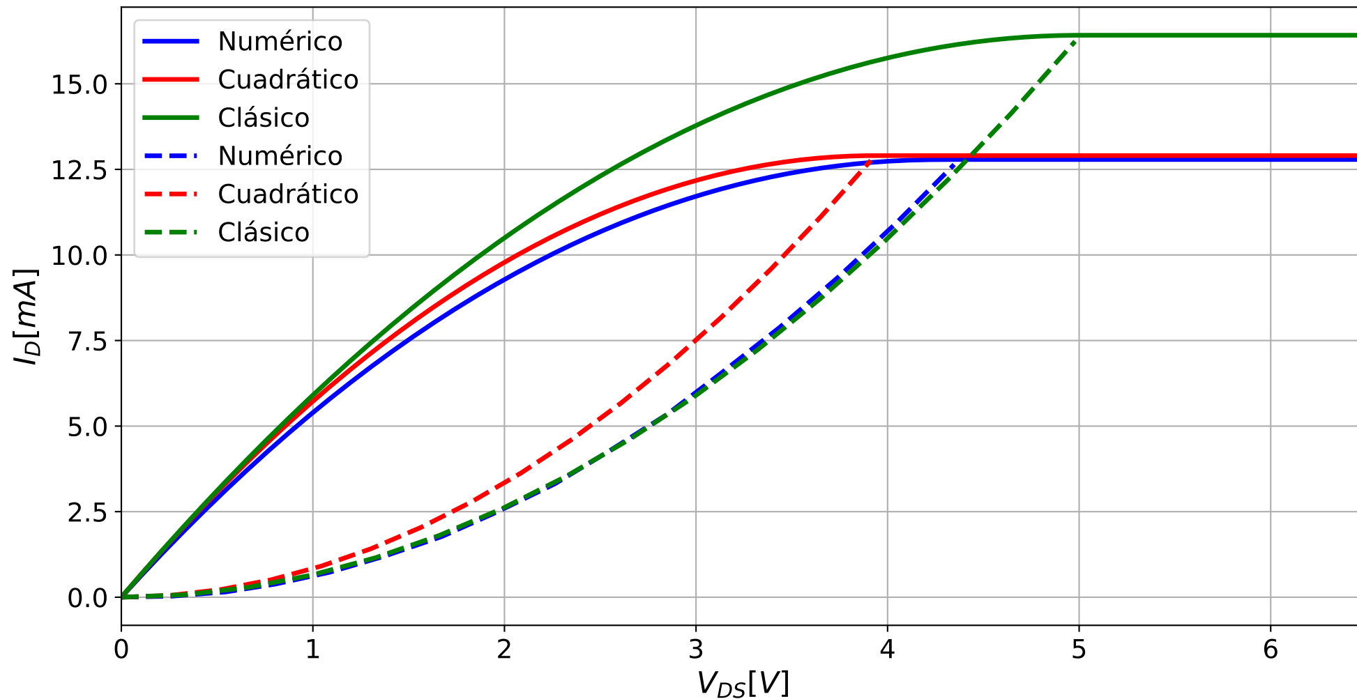
Curvas de salida para V_{GS} = 0,8 \cdot V_{DD} = 5.2 \text{ V}
